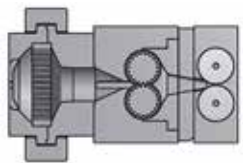
TRF 两辊喂料装置
