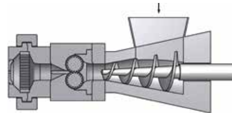
DSE 锥形双螺杆喂料装置
