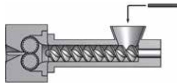
SF 螺杆喂料装置
